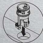
EZ CONX™ Top Mount bracket Support de montage supérieur EZ ConX™
